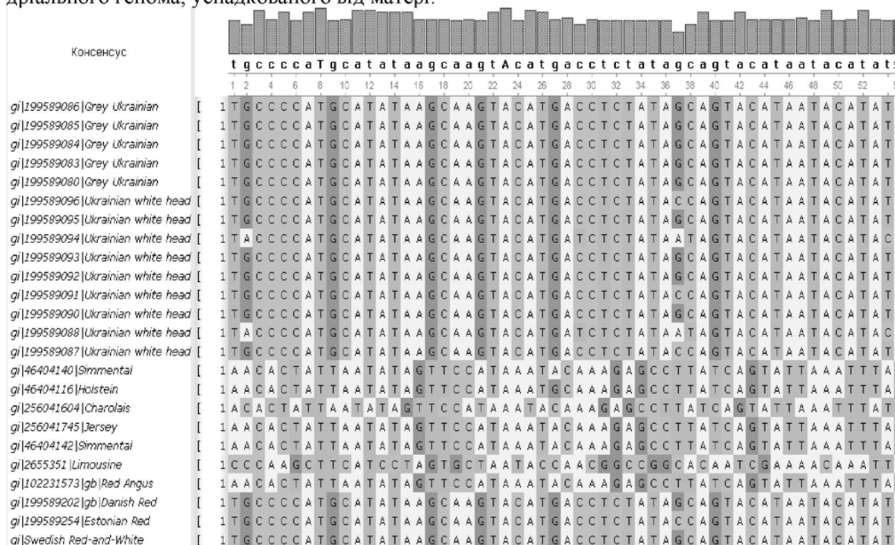
Рис. 1. Однонуклеотидний поліморфізм мітохондріальної ДНК за результатами локального вирівнювання послідовностей мтДНК тварин різних порід великої рогатої худоби (за даними GenBank, алгоритм ClustalW)
